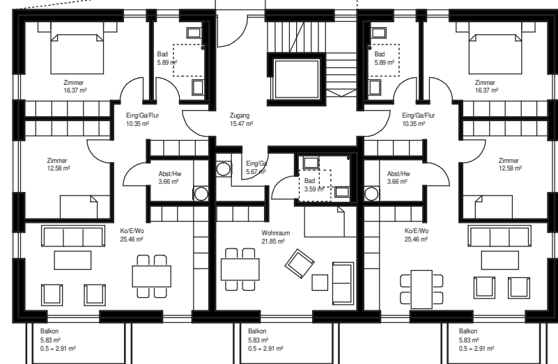
Erdgeschoss M 1:100
